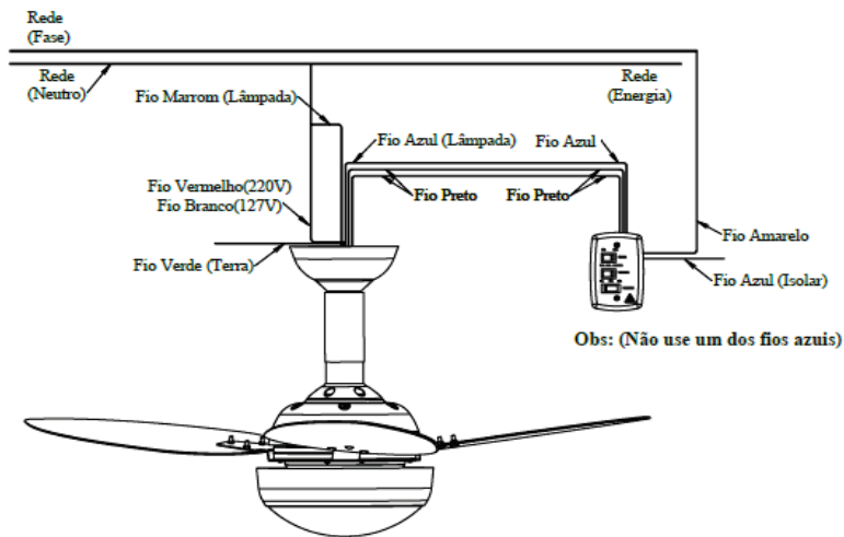
Ligação com Interruptor Simples
