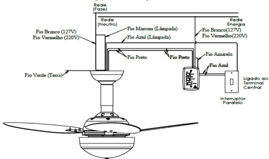
Ligação com Interruptor Paralelo
